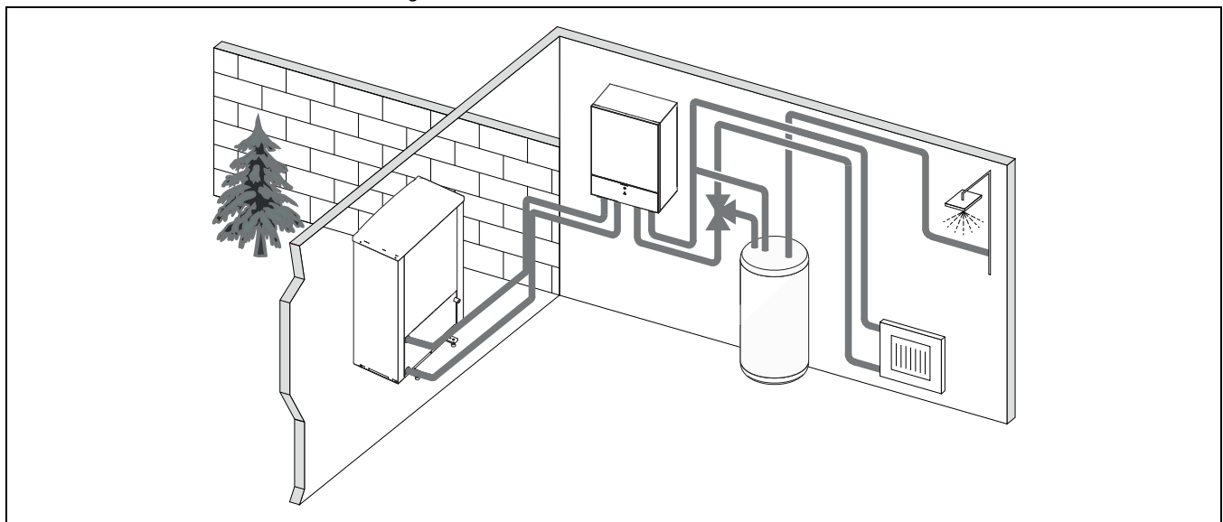
Joon. 3 Soojuspump Compress 7000i AW, siseüksus AWE elektrilise lisakütteseadme ja välise boileriga
