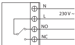
Ruumitermostaat, WT-T
