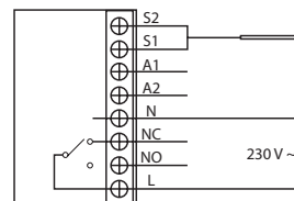
Ruumitermostaat, WT-DR/PR
