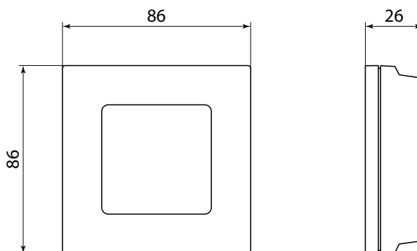
Danfoss Icon™ juhtmevaba ruumitermostaat
