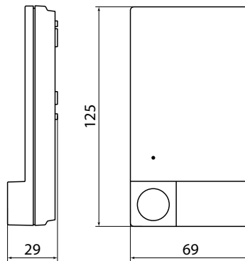
Danfoss Icon™ rakendusemoodul 088U1101
