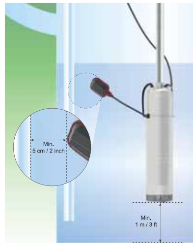
Joonis 3 SB HF pumba minimaalne ruum. See näide näitab paigaldamist kaevu
