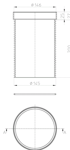
Schnitt A-A
