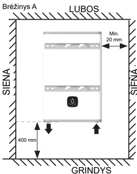
Karšto vandens išvadas turi būtivandens šildytuvo kairėje.
